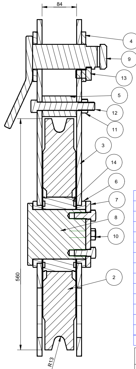
Section A-A
